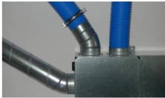
Abbildung 30: alle Anschlüsse für Spiro- und Kunststoffrohre DN 125
