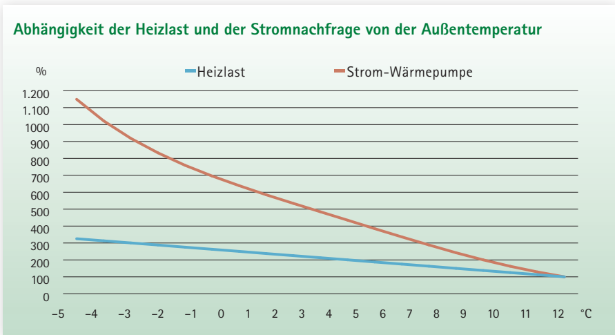
Abb. 2: Indexentwicklung der Heizlast und Leistungsnachfrage nach der Luftwärmepumpe in Abhängigkeit von der Außentemperatur (Index 100 % bei 12 Grad Celsius)
