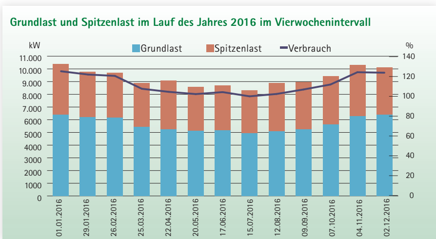
Abb. 1: Maximale und minimale Leistungswerte von jeweils 28 aufeinander folgenden Tagen beginnend vom angegebenen Startdatum – Kurve zeigt Verteilung der Nachfrage (kWh), niedrigster Vierwochenverbrauch auf 100 % gesetzt
